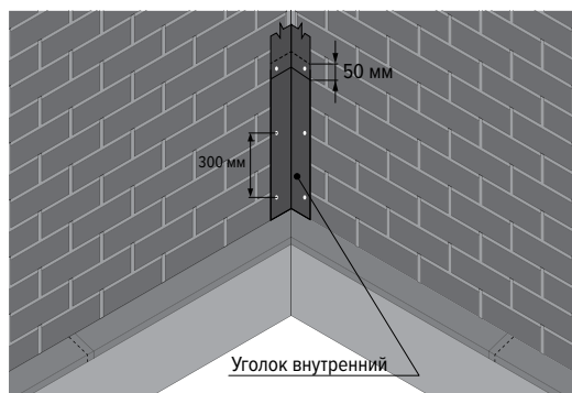
Рис. 12. Устройство внутренних углов
