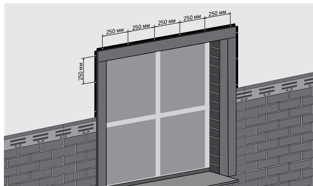
Рис. 23. Установка подоконного отлива
