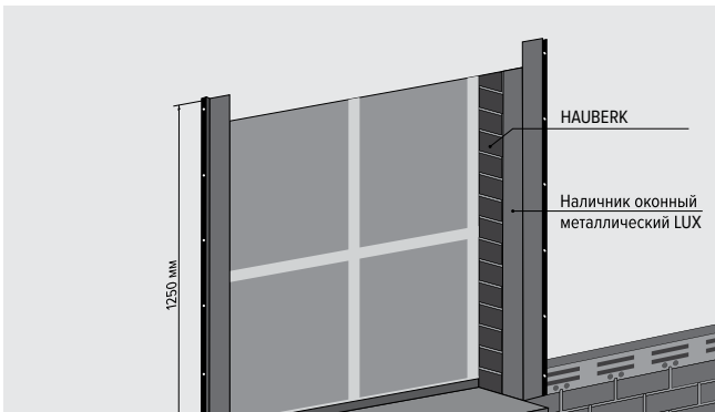
Рис. 22. Монтаж фасадной плитки вокруг оконных проемов
