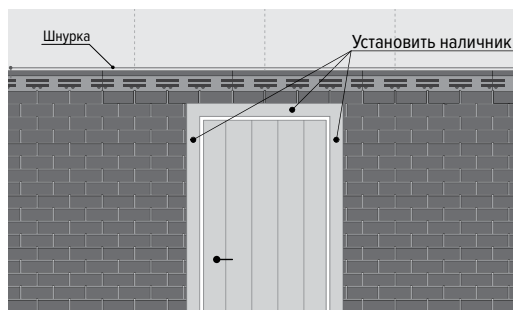
Рис. 14. Установка наличников
