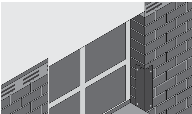
Рис. 17. Монтаж оконного наличника сбоку проема
