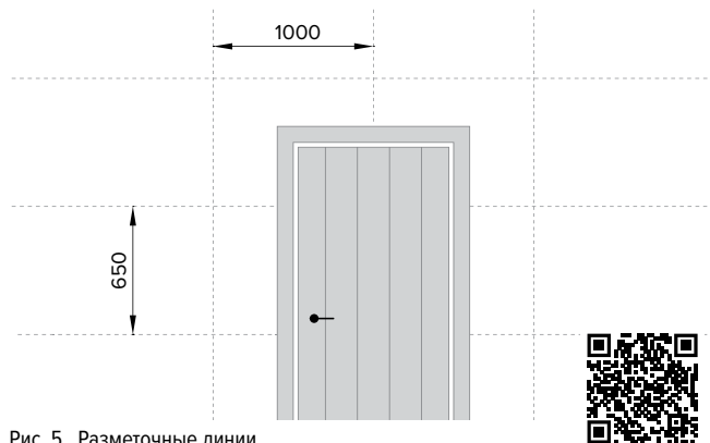
Рис. 5. Разметочные линии
