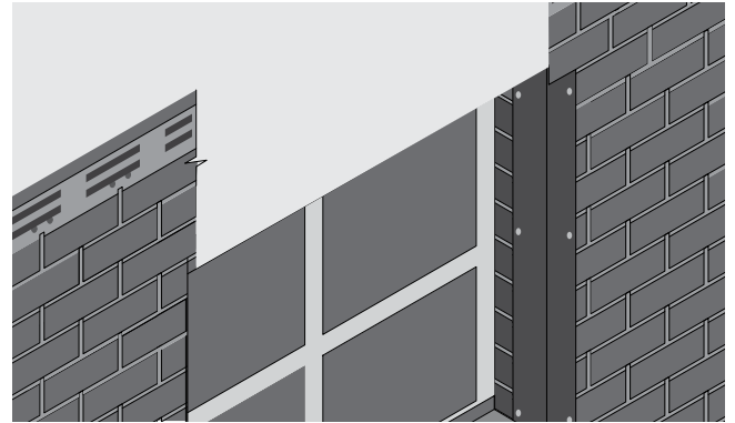
Рис. 18. Монтаж бокового наличника (верхний край заходит под фасадную плитку)
