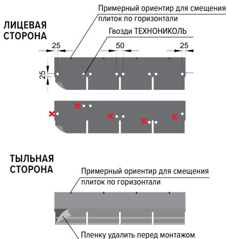
Рис. 2.2. Схема крепления фасадной плитки на 8 гвоздей
