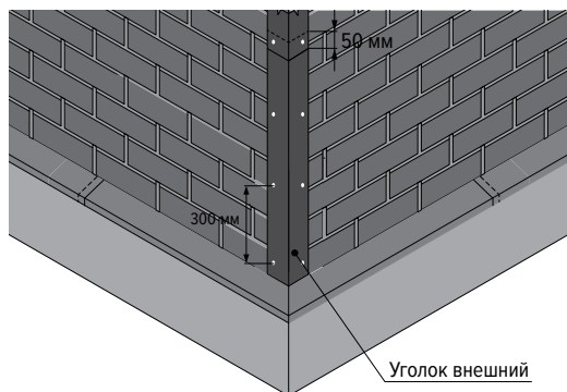
Рис. 11. Устройство внешних углов
