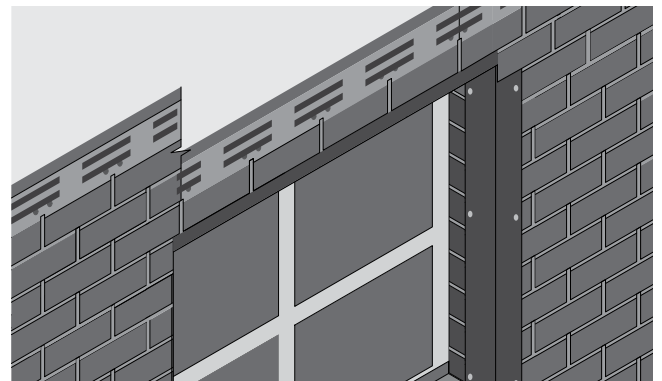
Рис. 20. Монтаж фасадной плитки поверх оконного наличника сверху проема
