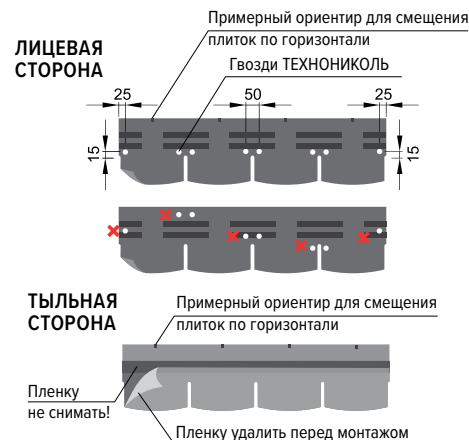
Рис. 2.1. Схема крепления фасадной плитки на 8 гвоздей
