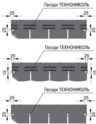
Рис. 3. Схема крепления фасадной плитки на 5 гвоздей
