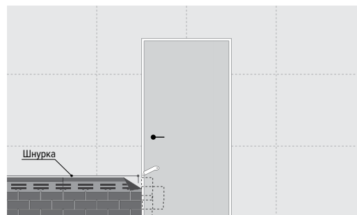
Рис. 13. Монтаж фасадной плитки вокруг дверных проемов
