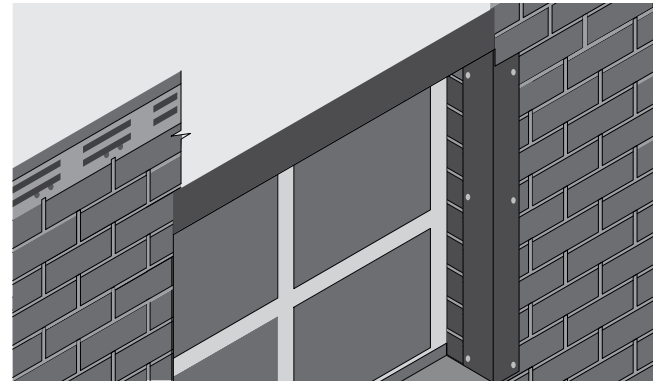
Рис. 19. Монтаж оконного наличника сверху проема
