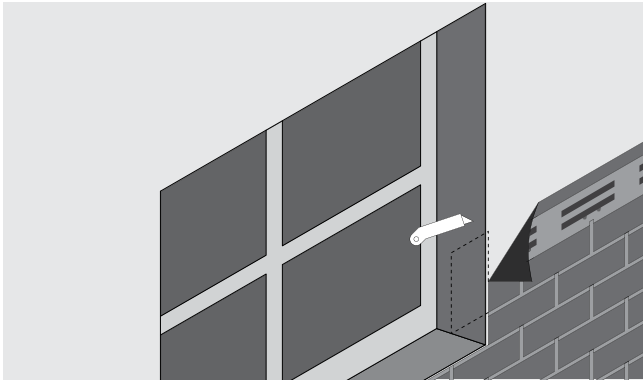
Рис. 15. Монтаж фасадной плитки вокруг оконных проемов
